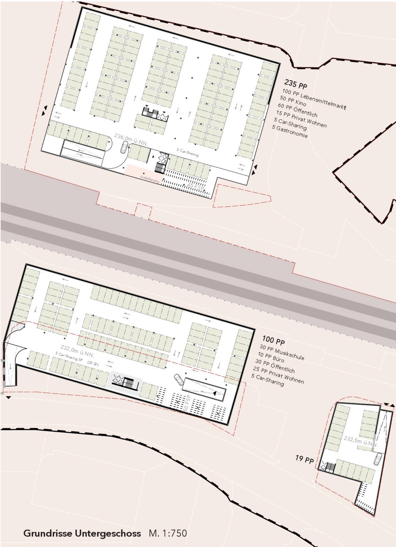
Grundrisse Untergeschoss M. 1:750
