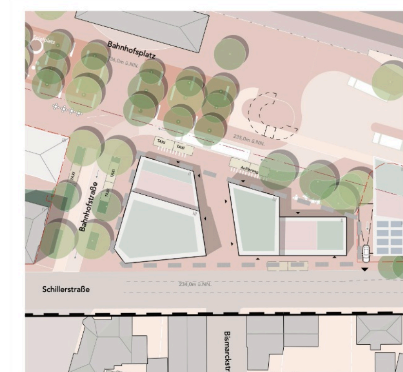
Dachaufsicht
