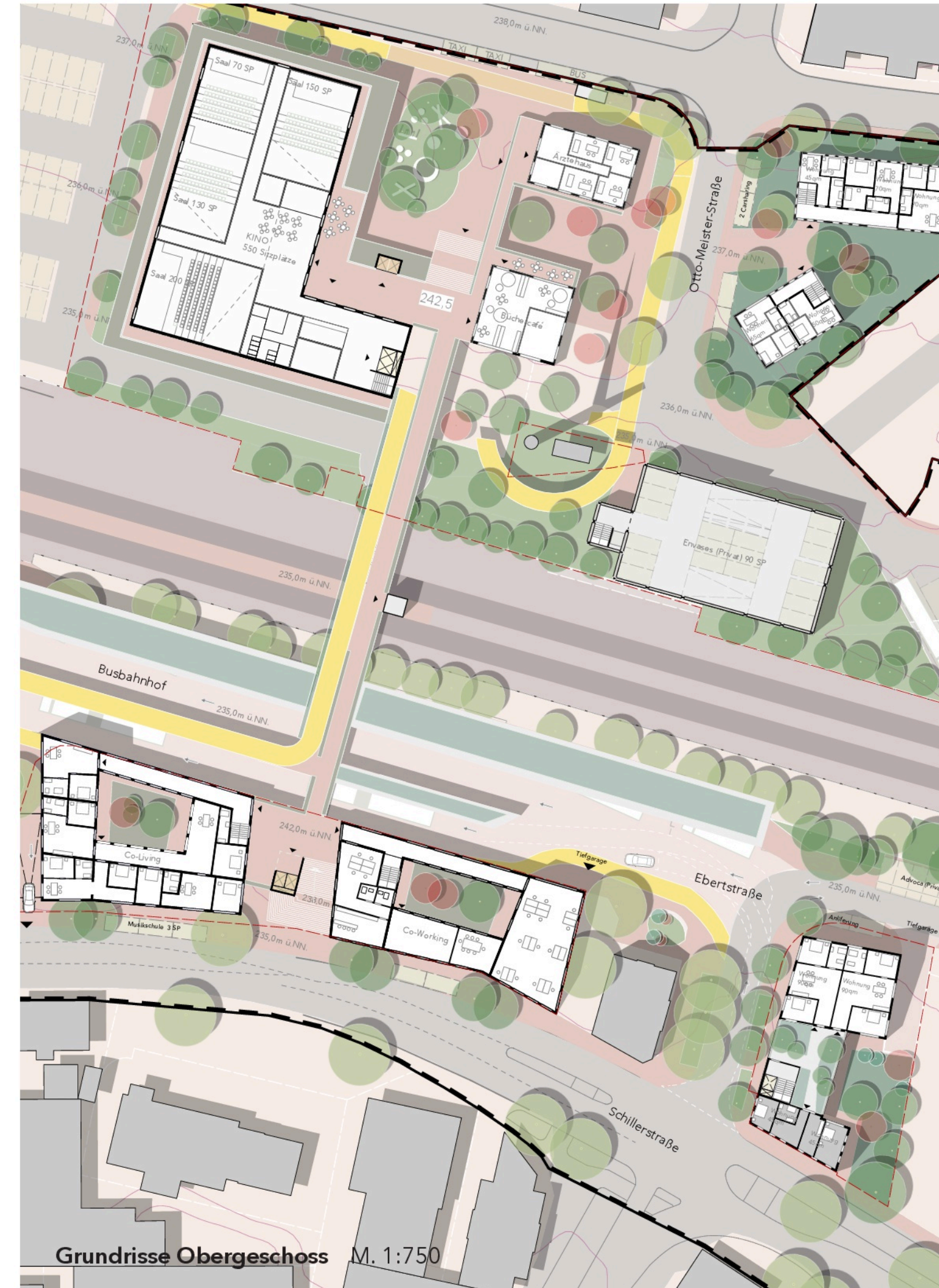
Grundrisse Obergeschoss M. 1:750
